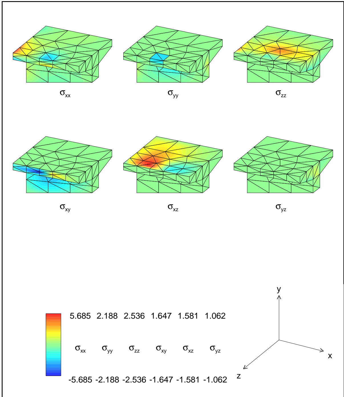
Figura 13.2 - Tensões obtidas com elementos de equilíbrio de grau três.
