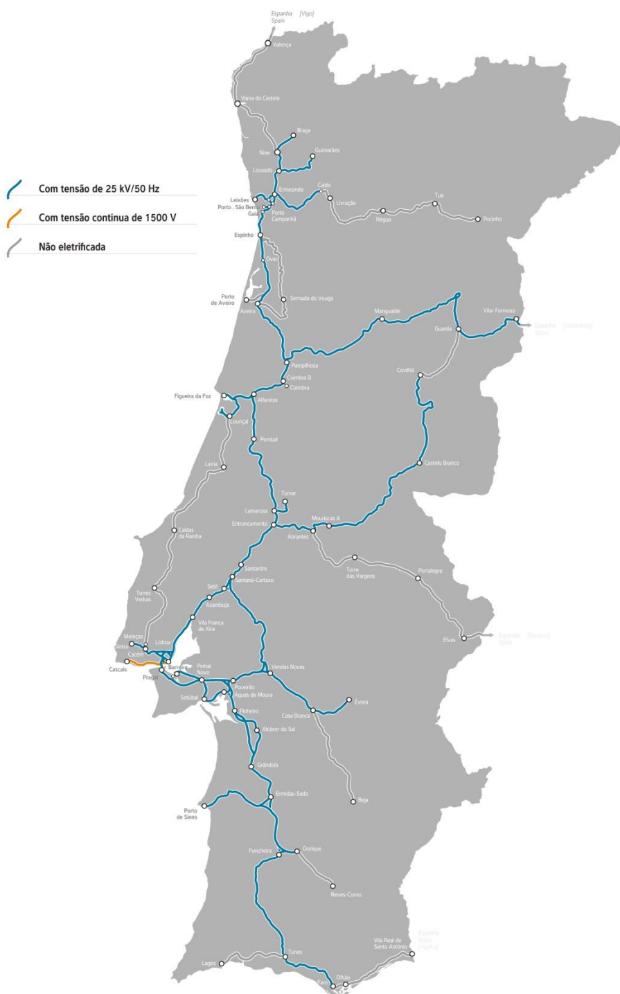
Ilustração 54 - Características da rede ferroviária nacional em 2013 - Electrificação
