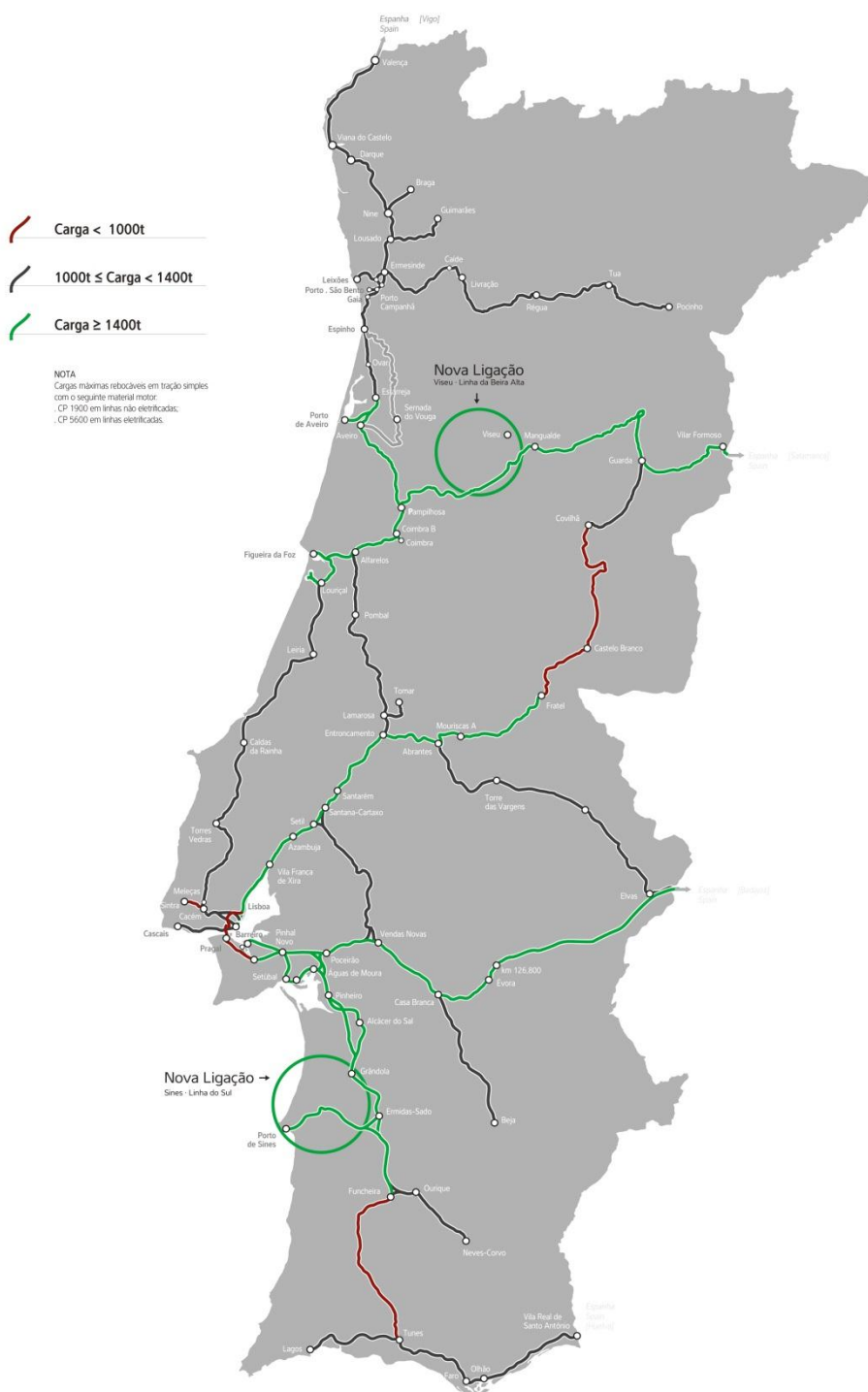
Ilustração 53 - Características da rede ferroviária nacional em 2020/22 - Cargas máximas
