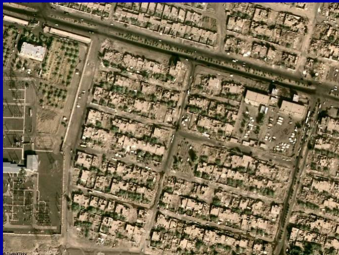
Sismo de Bam (Irão, 2003) – Vista de satélite
