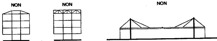
c) structures suspendues : à éviter
