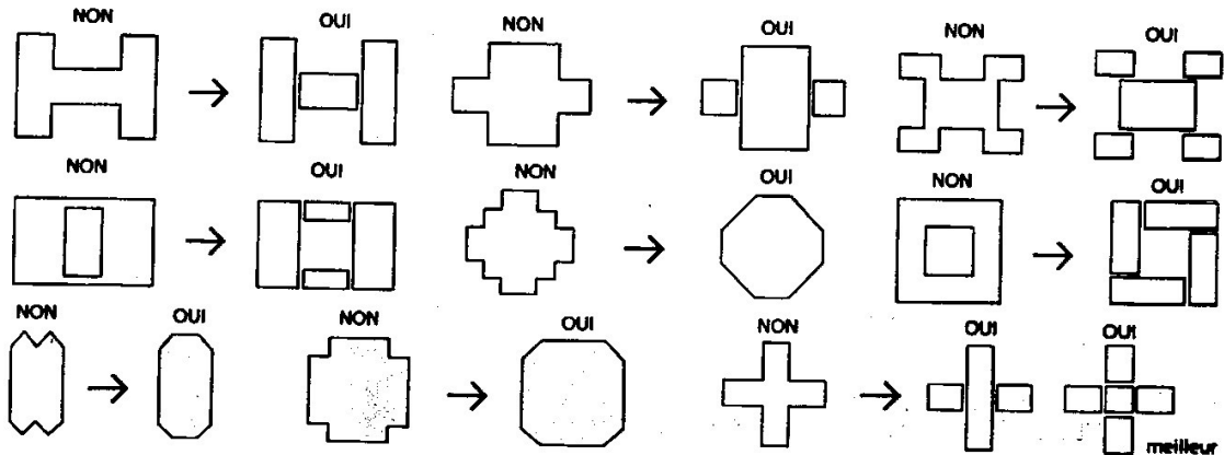
plan complexe à 2 axes de symétrie
