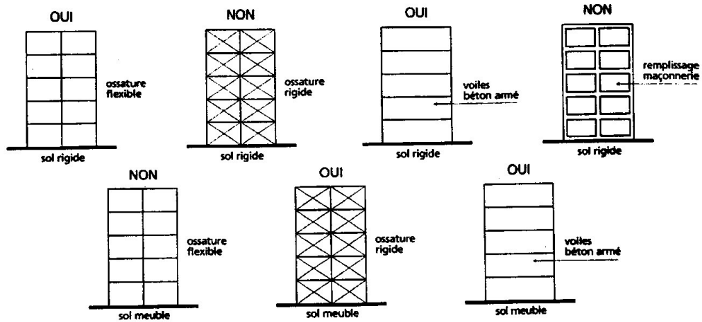
a) prise en compte de la nature du sol
